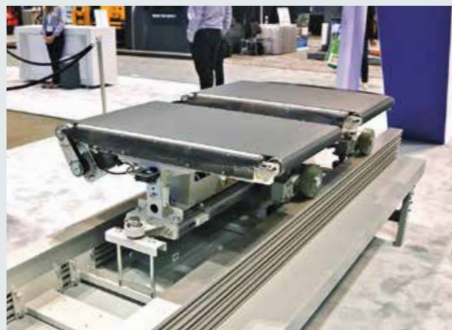
高速仕分けシステム「クロスベルトソーター」の一部を展示。
