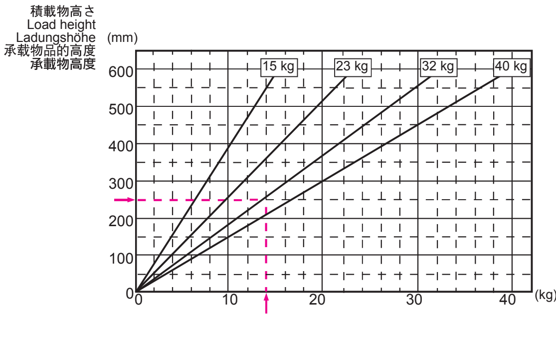
圖一 LVC-04C5 的最大荷重選定表
